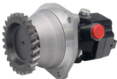
POMPA INIEZIONE Injection Pump
