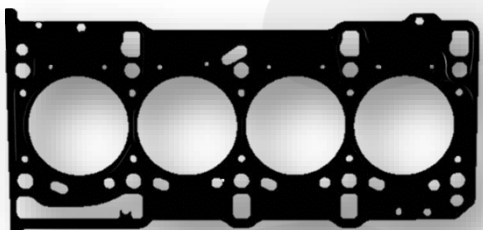
Guarnizione TESTA – 1 tacca Head gasket – with 1 hole
